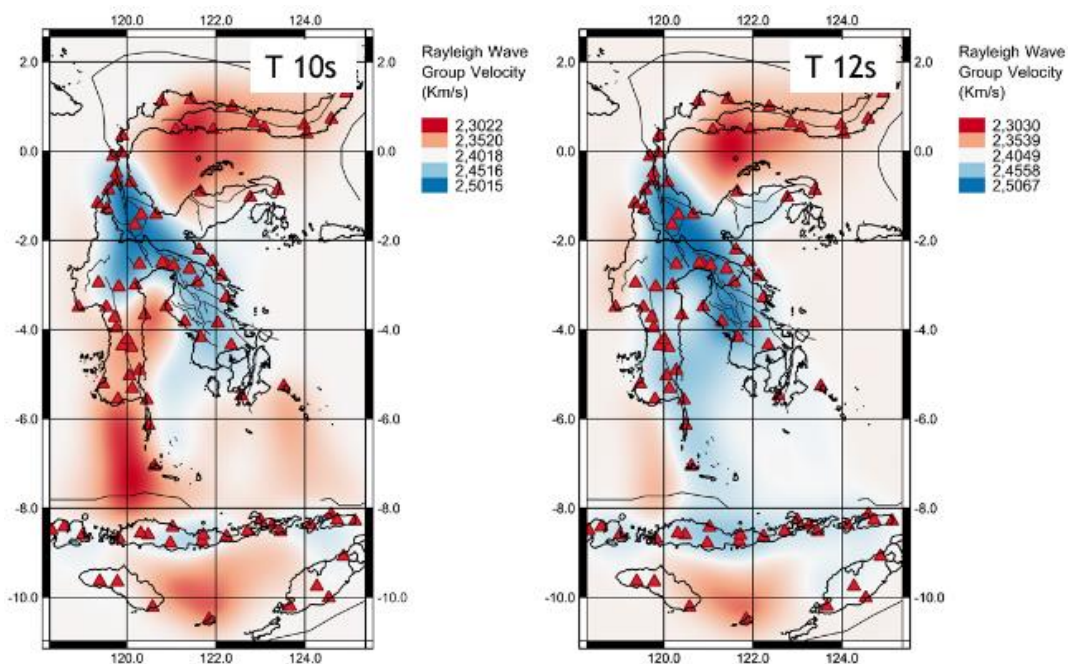
Gambar 10. Peta kecepatan group gelombang Rayleigh periode 10 dan 12 s di Pulau Sulawesi dan NTT (segitiga merah merupakan stasiun seismik dan garis hitam merupakan patahan).
