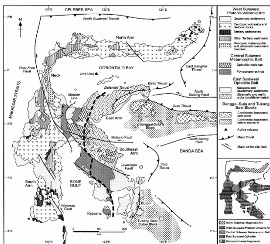
Gambar 7. Peta Geologi Sulawesi [12].
